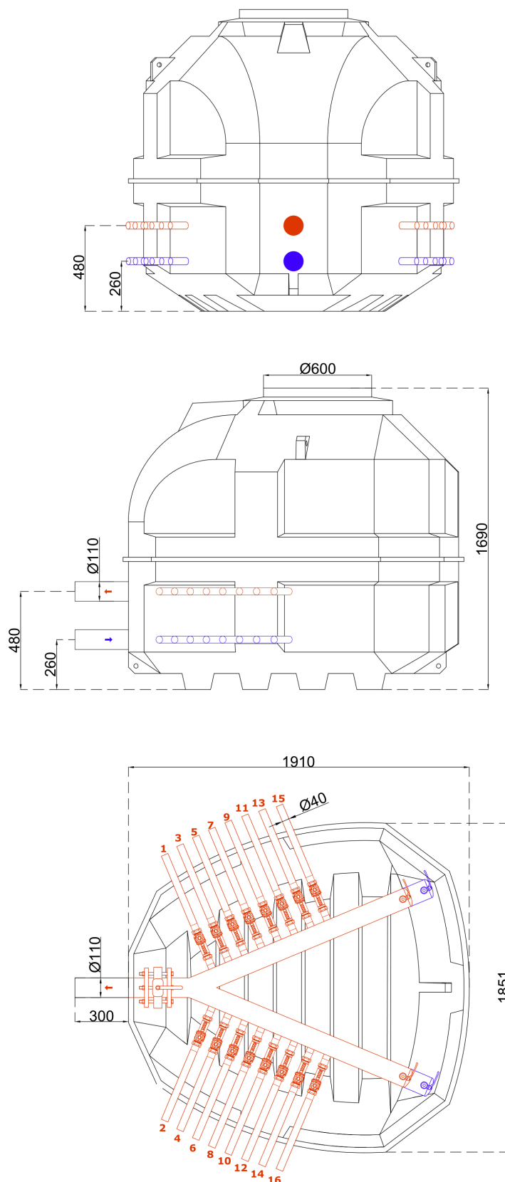
Rys. 5. Studnia Terra V-SERIES z rotametrami - 16 sekcji
