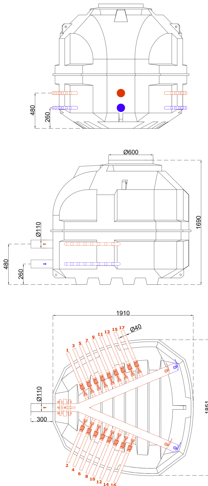
Rys. 6. Studnia Terra V-SERIES z rotametrami – 17 sekcji
