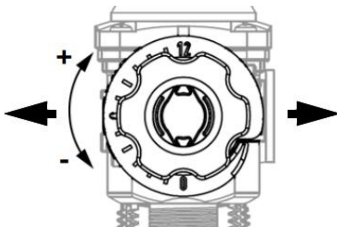
Rys. 25. Pokrętło rotametu tworzywowego
