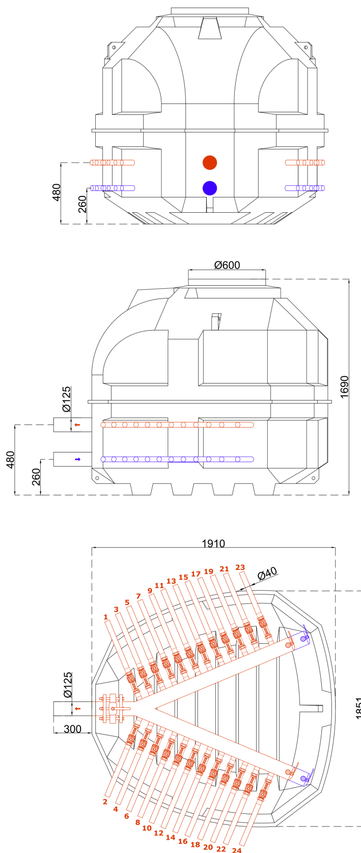
Rys. 13. Studnia Terra V-SERIES z rotametrami – 24 sekcje
