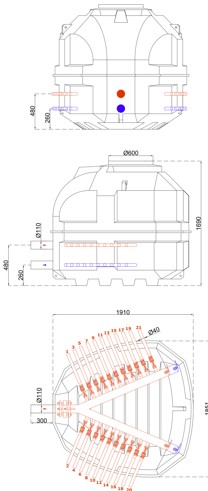
Rys. 10. Studnia Terra V-SERIES z rotametrami - 21 sekcji
