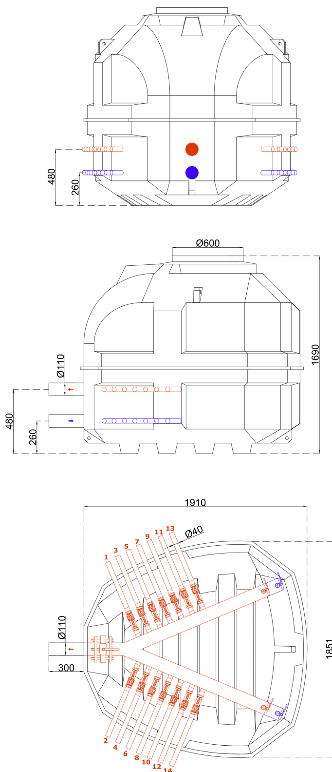
Rys. 3. Studnia Terra V-SERIES z rotametrami - 14 sekcji
