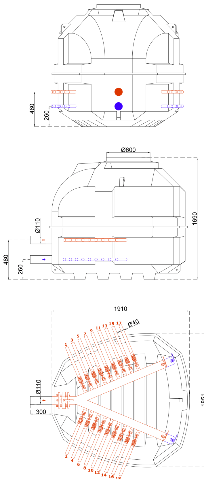
Rys. 7. Studnia Terra V-SERIES z rotametrami - 18 sekcji
