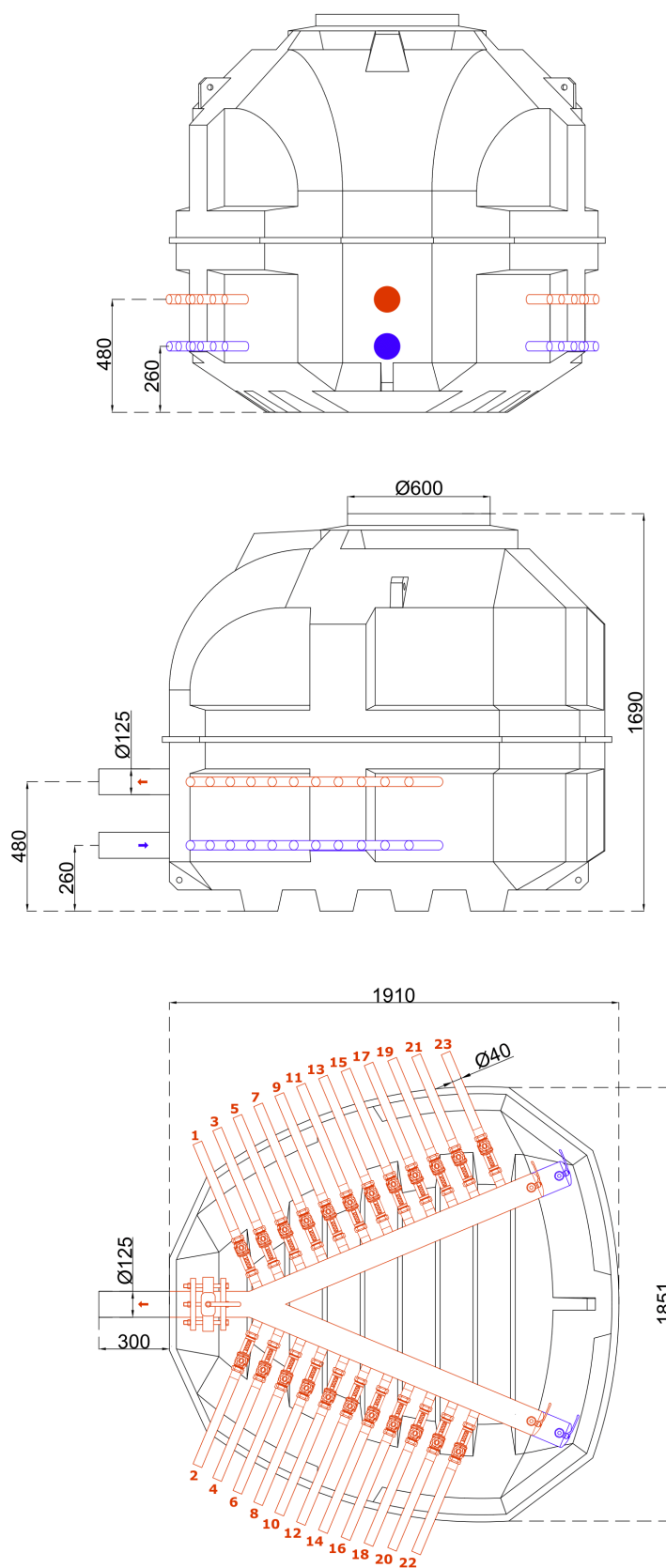
Rys. 12. Studnia Terra V-SERIES z rotametrami - 23 sekcje
