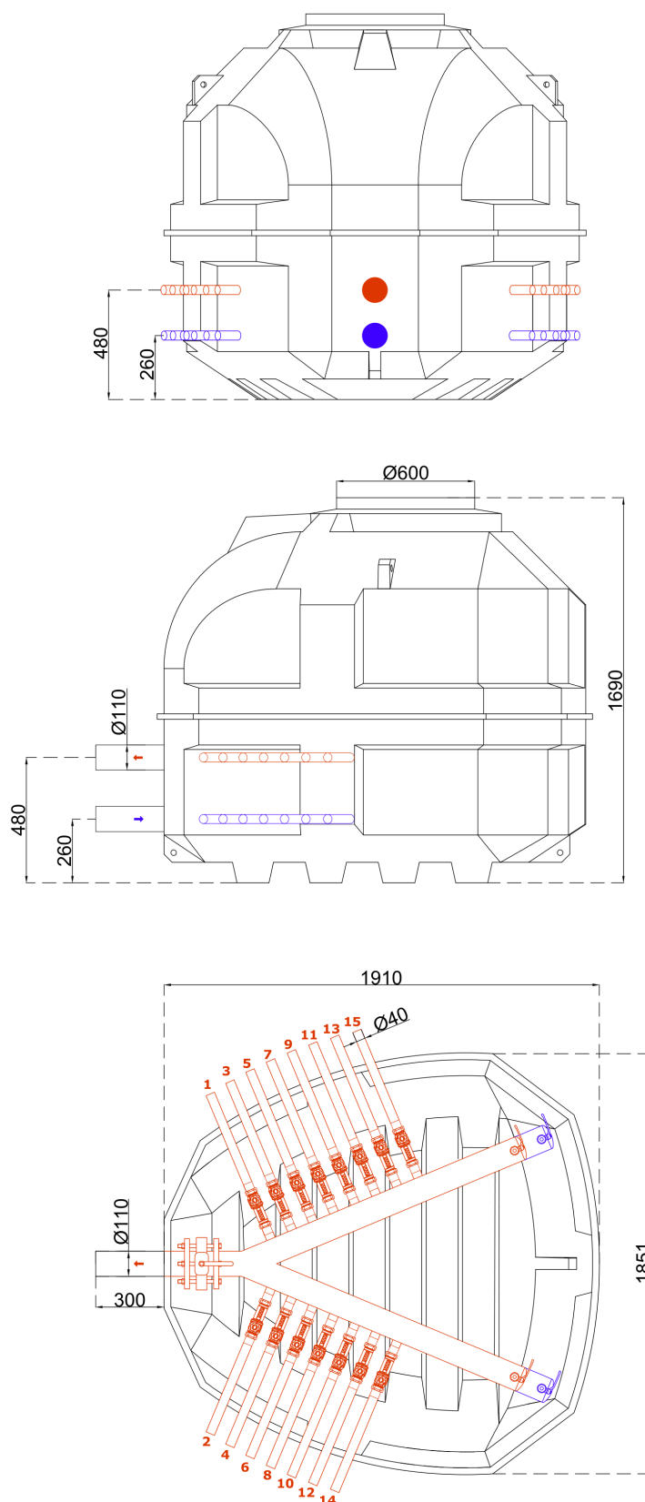
Rys. 4. Studnia Terra V-SERIES z rotametrami - 15 sekcji
