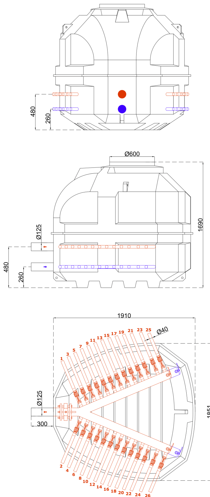
Rys. 15. Studnia Terra V-SERIES z rotametrami - 26 sekcji
