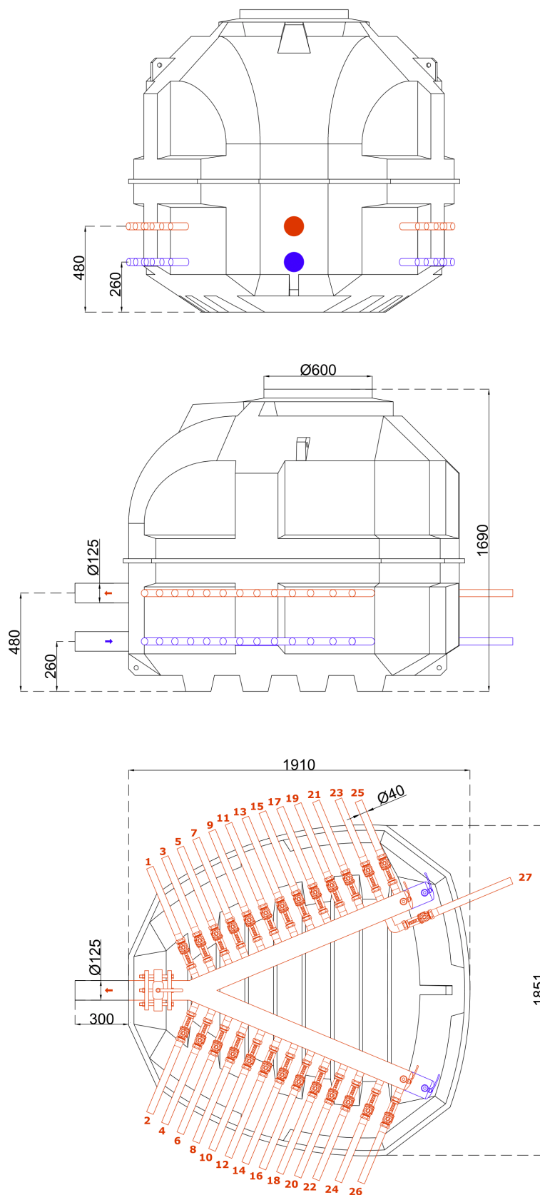
Rys. 16. Studnia Terra V-SERIES z rotametrami - 27 sekcji
