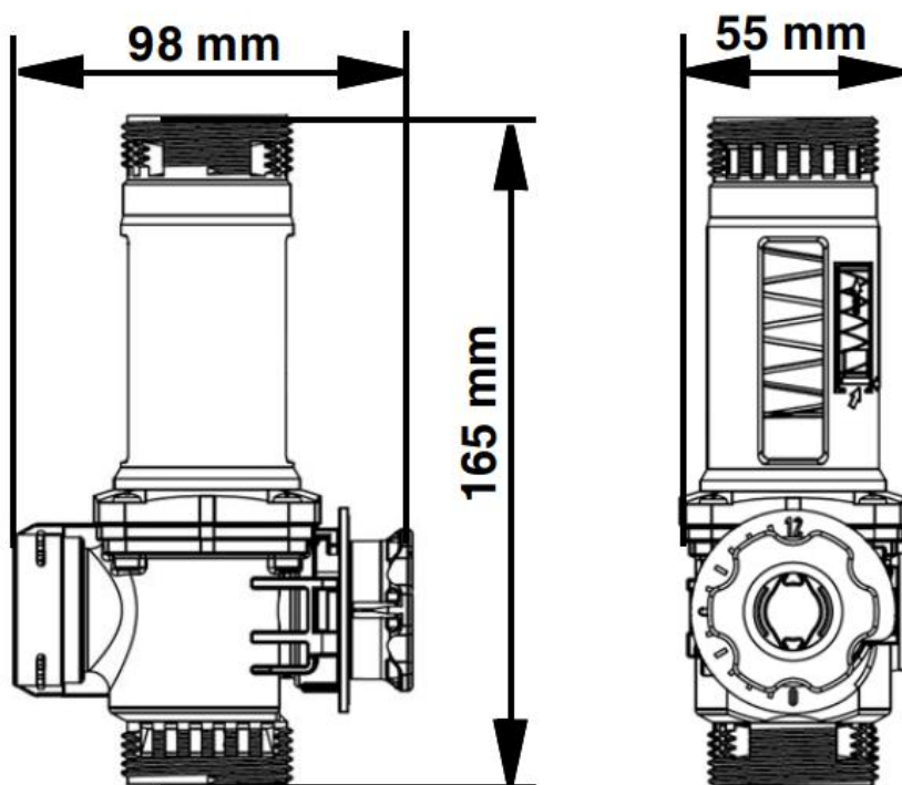
Rys. 23. Korpus przepływomierza liniowego PRAWTECH typu E: 5-42 l/min
