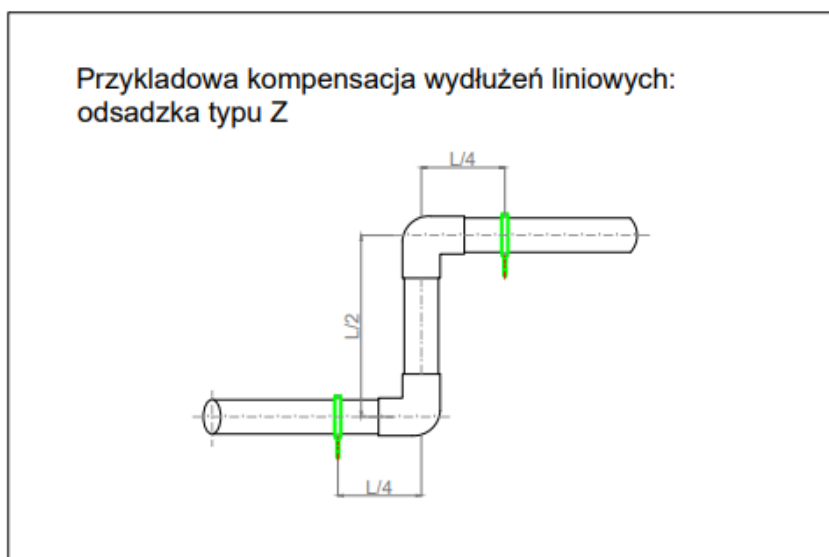
Rys. 21. Odsadzka typu Z
