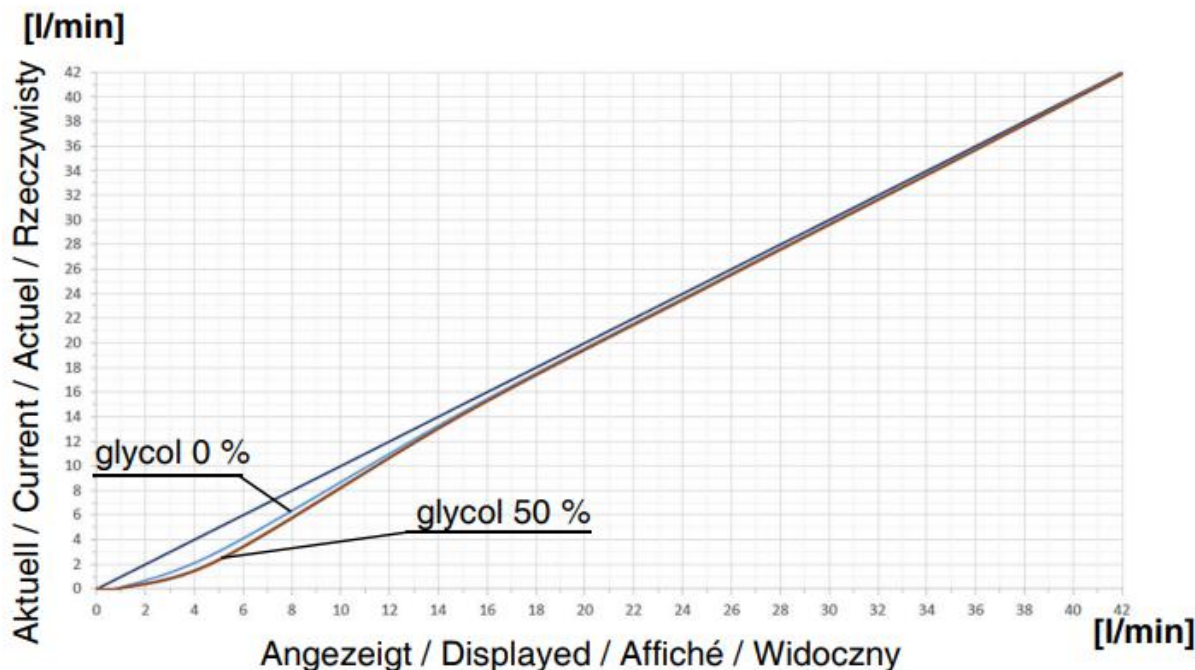
Rys. 27. Krzywe korekcyjne dla rotametrów tworzywowych
