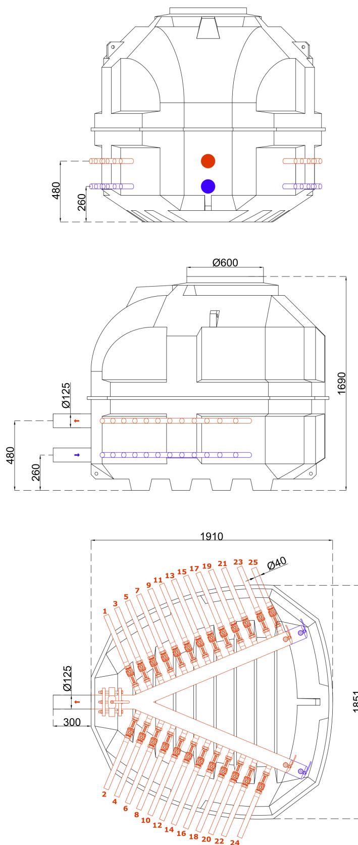
Rys. 14. Studnia Terra V-SERIES z rotametrami - 25 sekcji
