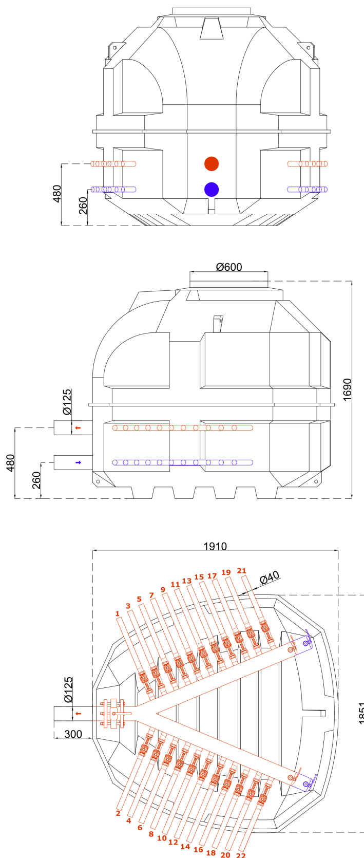
Rys. 11. Studnia Terra V-SERIES z rotametrami - 22 sekcje
