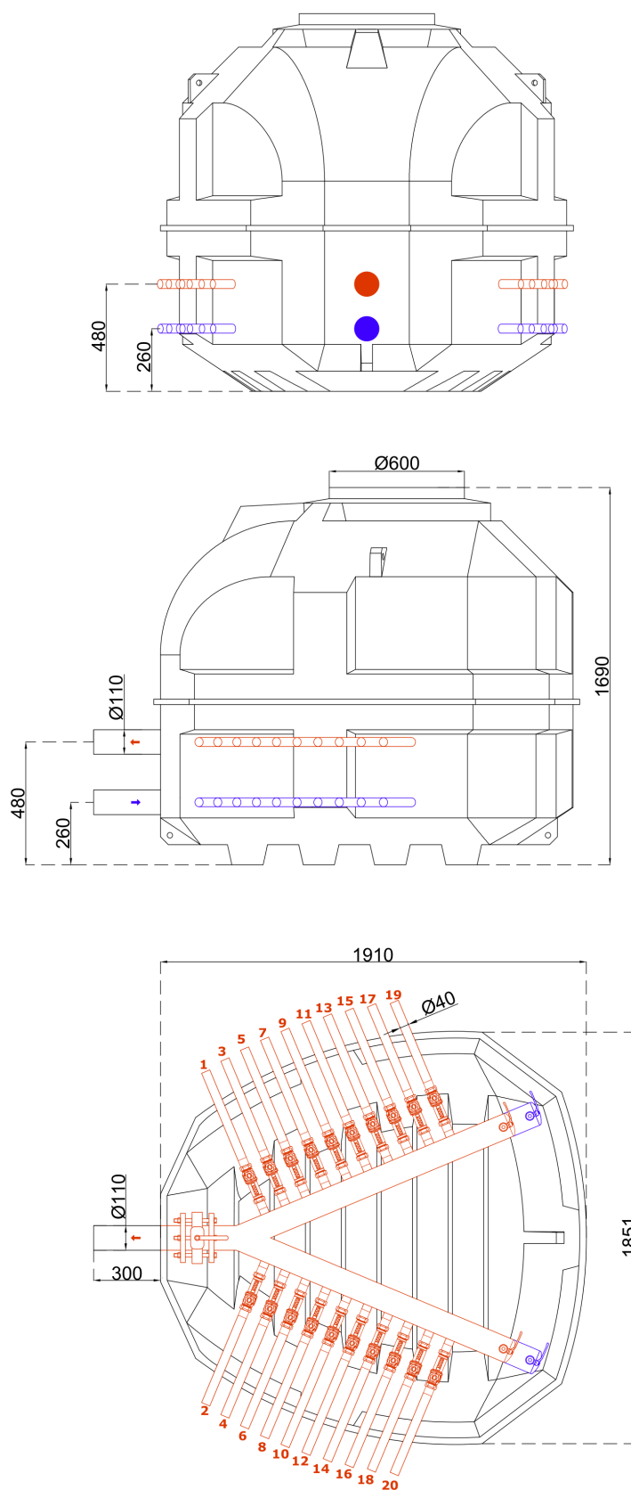
Rys. 9. Studnia Terra V-SERIES z rotametrami - 20 sekcji
