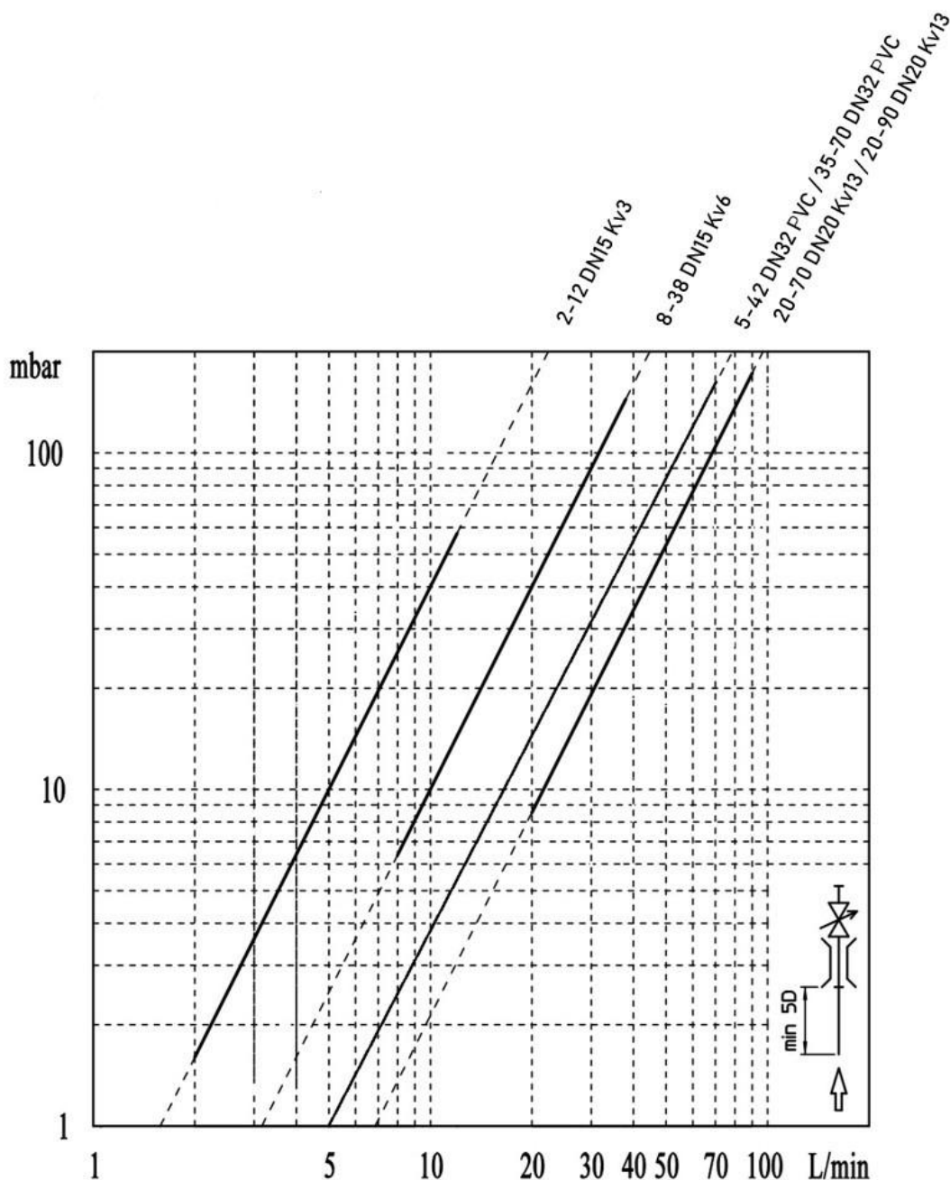
Rys. 26. Charakterystyka oporów hydraulicznych dla rotametrów w ofercie PRAWTECH
