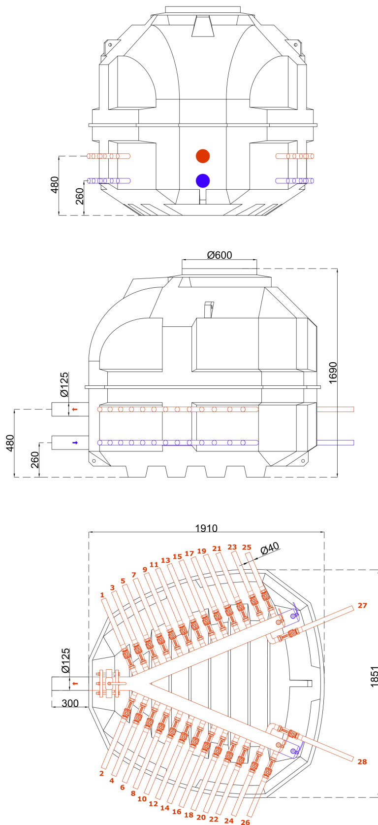
Rys. 17. Studnia Terra V-SERIES z rotametrami - 28 sekcji
