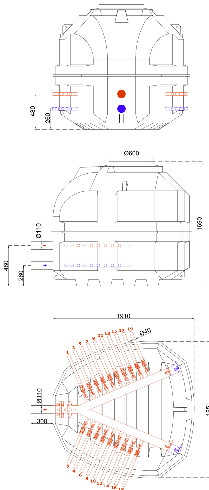
Rys. 8. Studnia Terra V-SERIES z rotametrami - 19 sekcji
