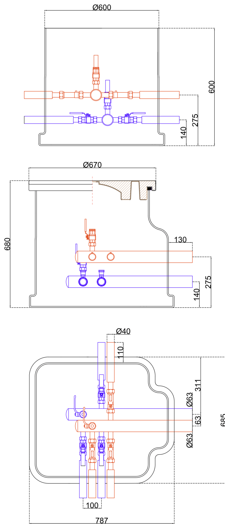
Rys. 4. Studnia Terra MINI z rotametrami - 3 sekcje
