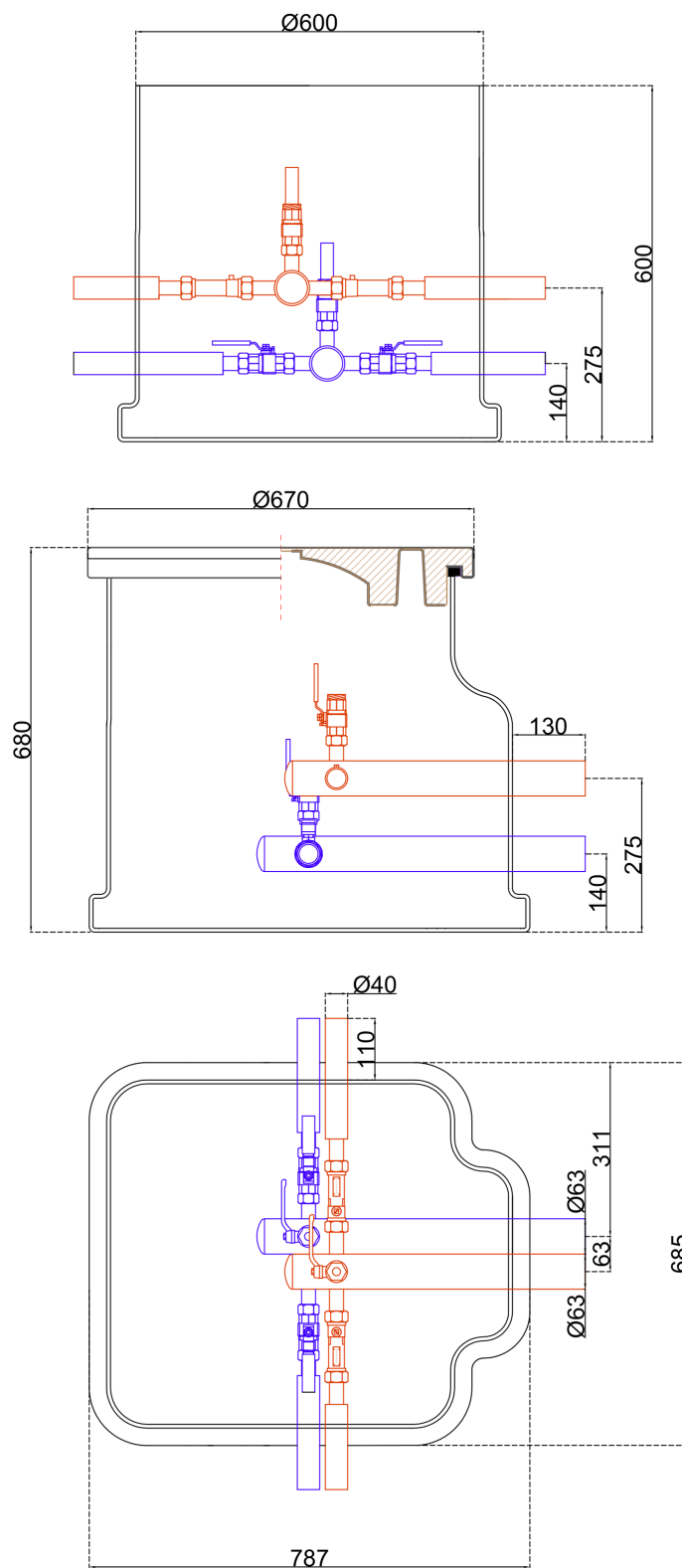
Rys. 3. Studnia Terra MINI z rotametrami - 2 sekcje
