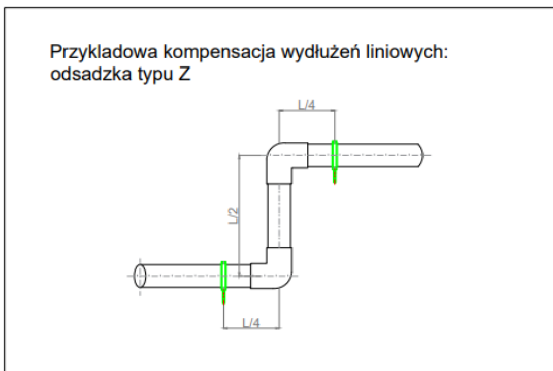
Rys. 11. Odsadzka typu Z
