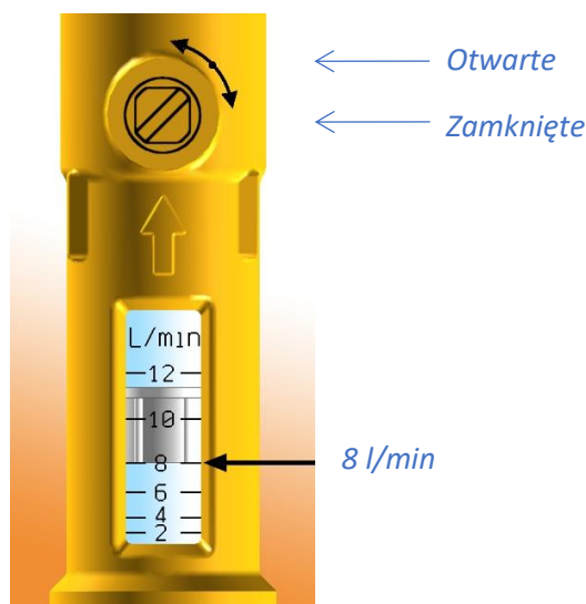
Rys. 12. Korpus przepływomierza liniowego PRAWTECH typu A: 2-12 l/min
