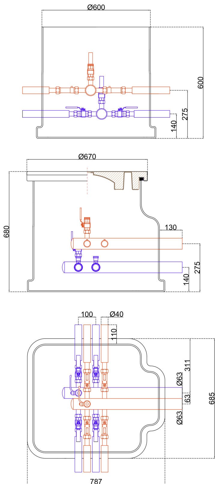
Rys. 5. Studnia Terra MINI z rotametrami - 4 sekcje
