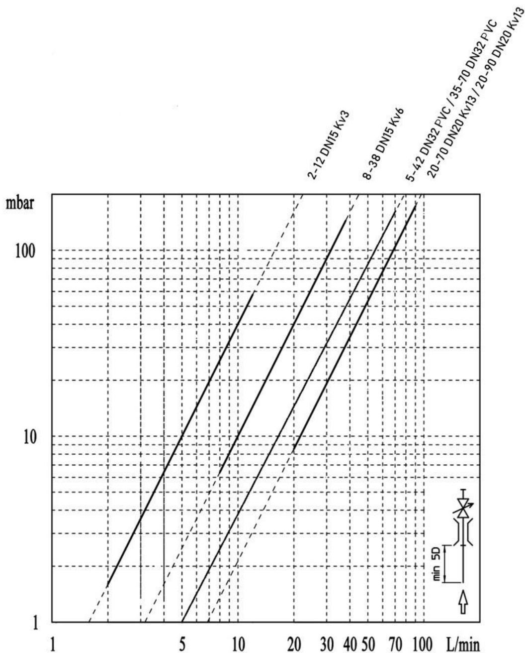
Rys. 14. Charakterystyka oporów hydraulicznych dla rotametrów w ofercie PRAWTECH
