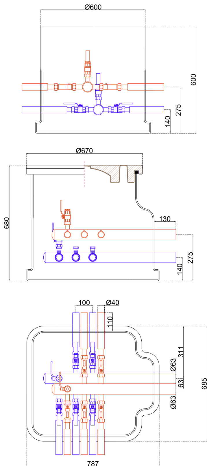
Rys. 6. Studnia Terra MINI z rotametrami - 5 sekcji
