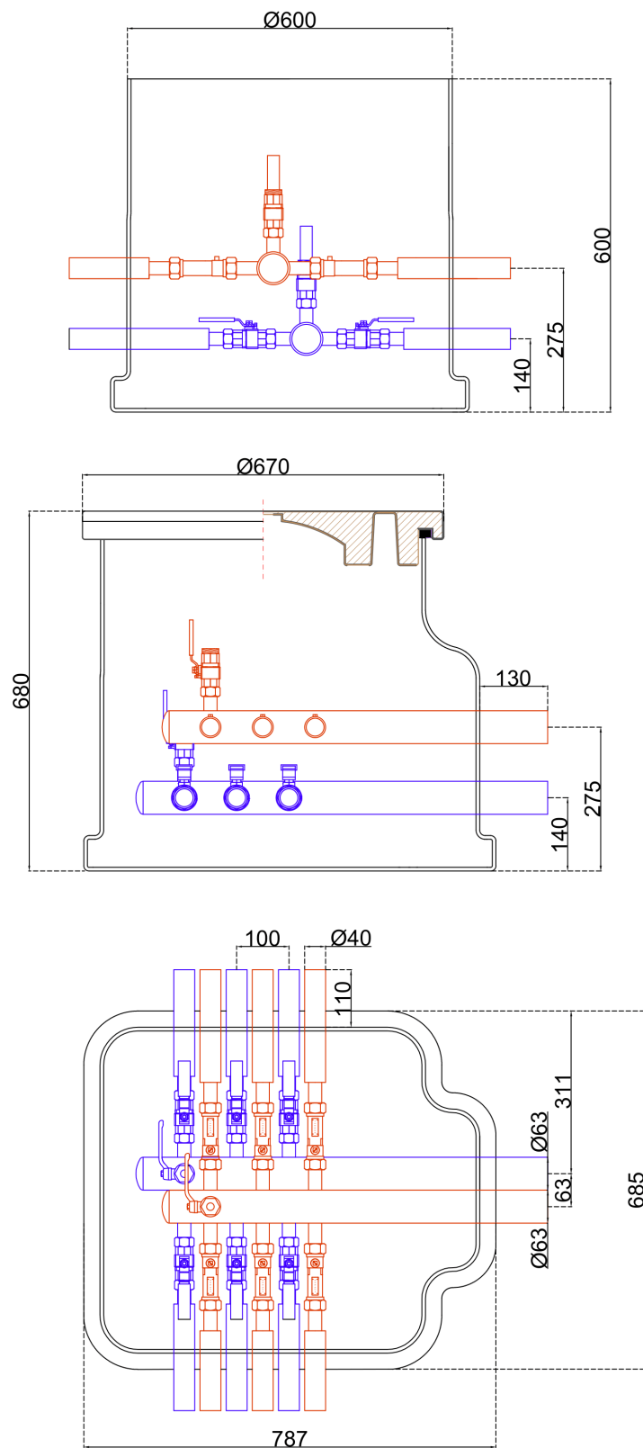
Rys. 7. Studnia Terra MINI z rotametrami - 6 sekcji
